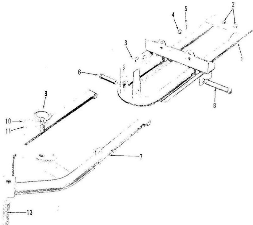
Fig. 2 - Dozer Frame - 19-80
